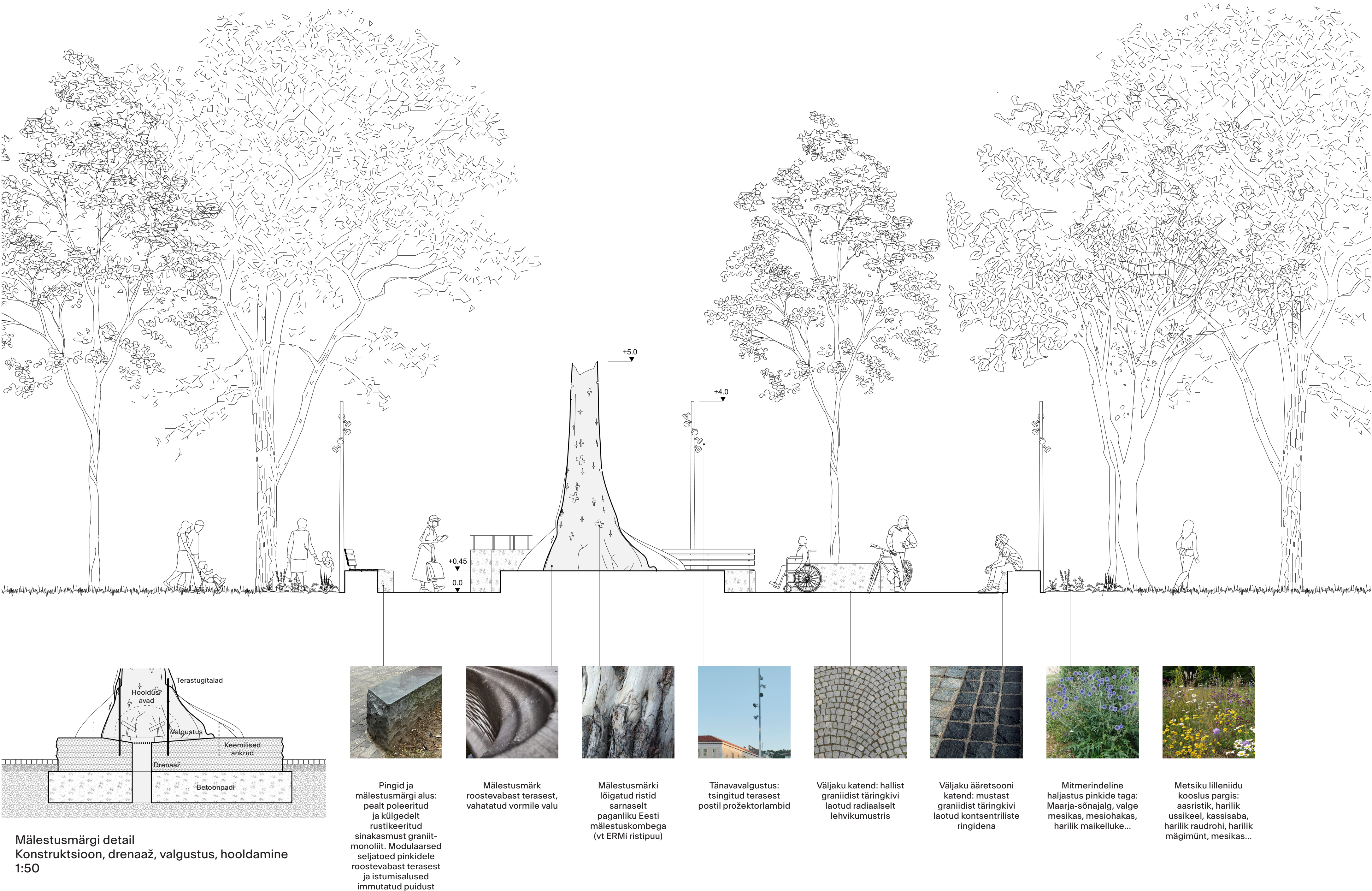
Lõige risti Jaama tänavaga 1:50
